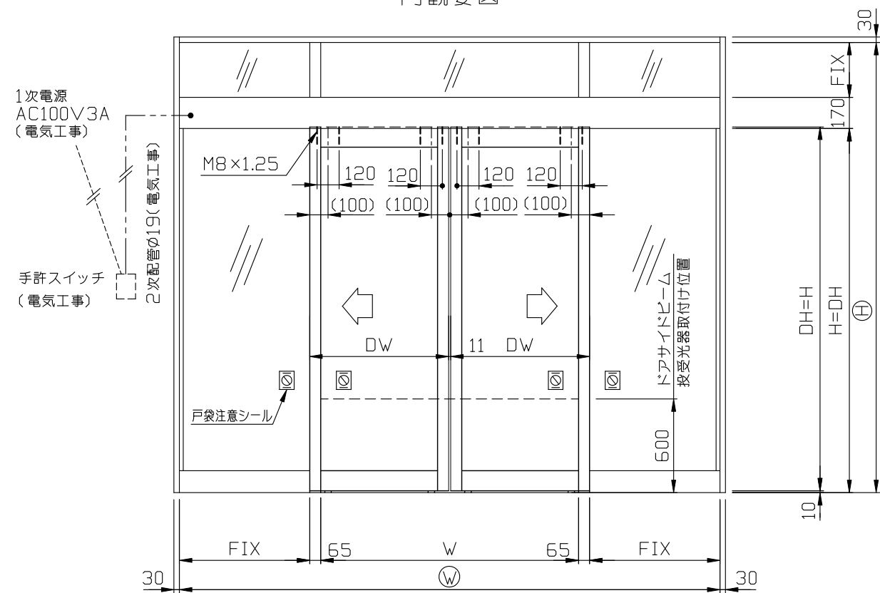
内観姿図
