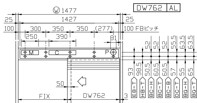
EBベースのフラットバー納り (参考例)
