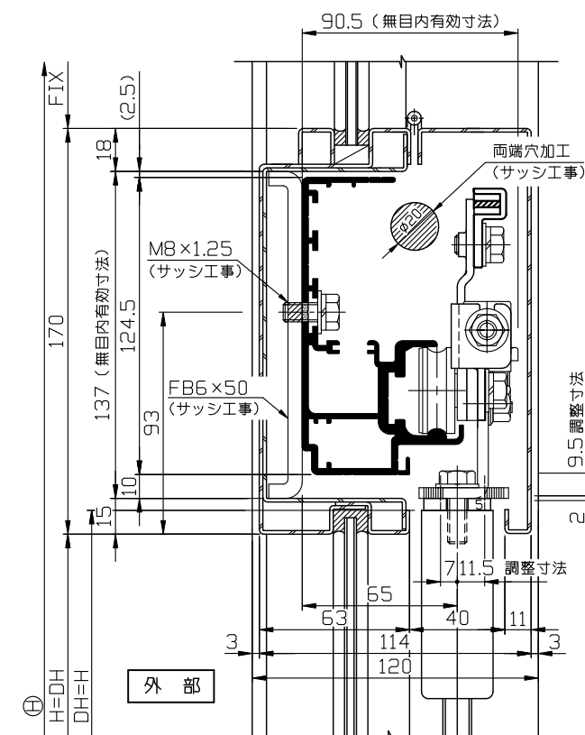
EBベースのフラットバー納り (参考例)
